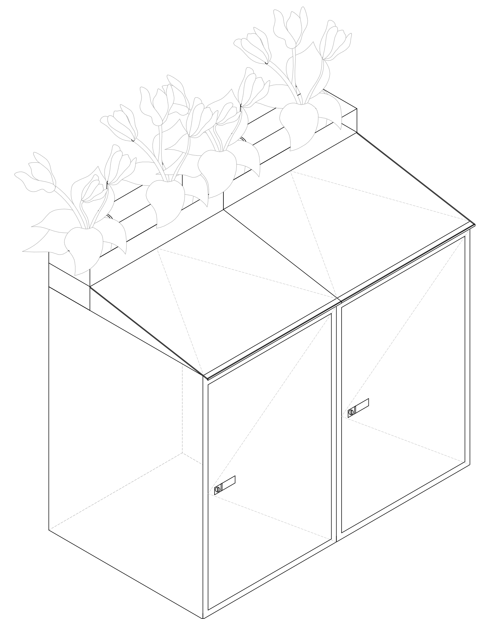
4 GARBAGE AXONOMETRIC SCALE: 1 1/2" = 1'-0"
