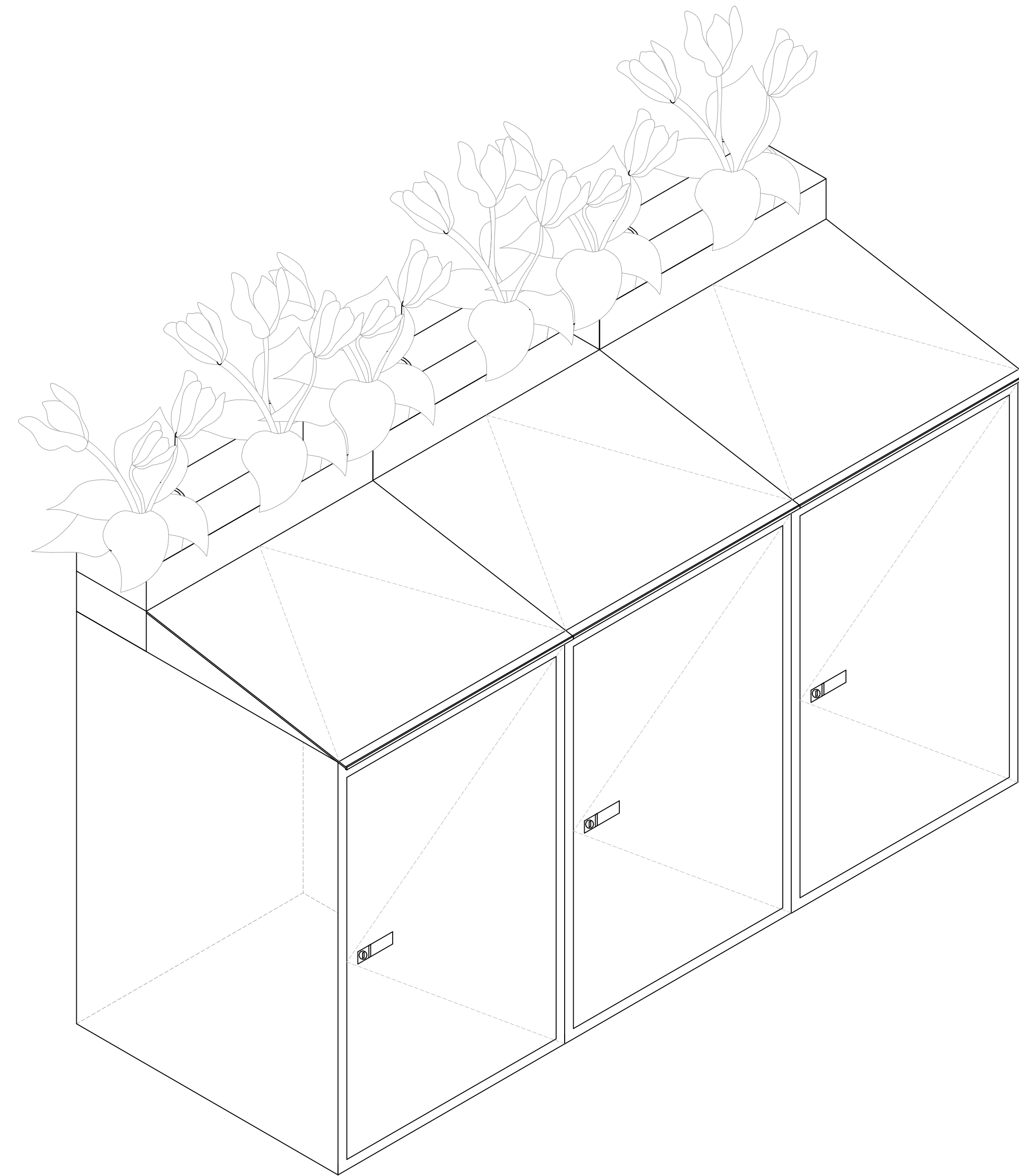
4 GARBAGE AXONOMETRIC SCALE: 1 1/2" = 1'-0"
