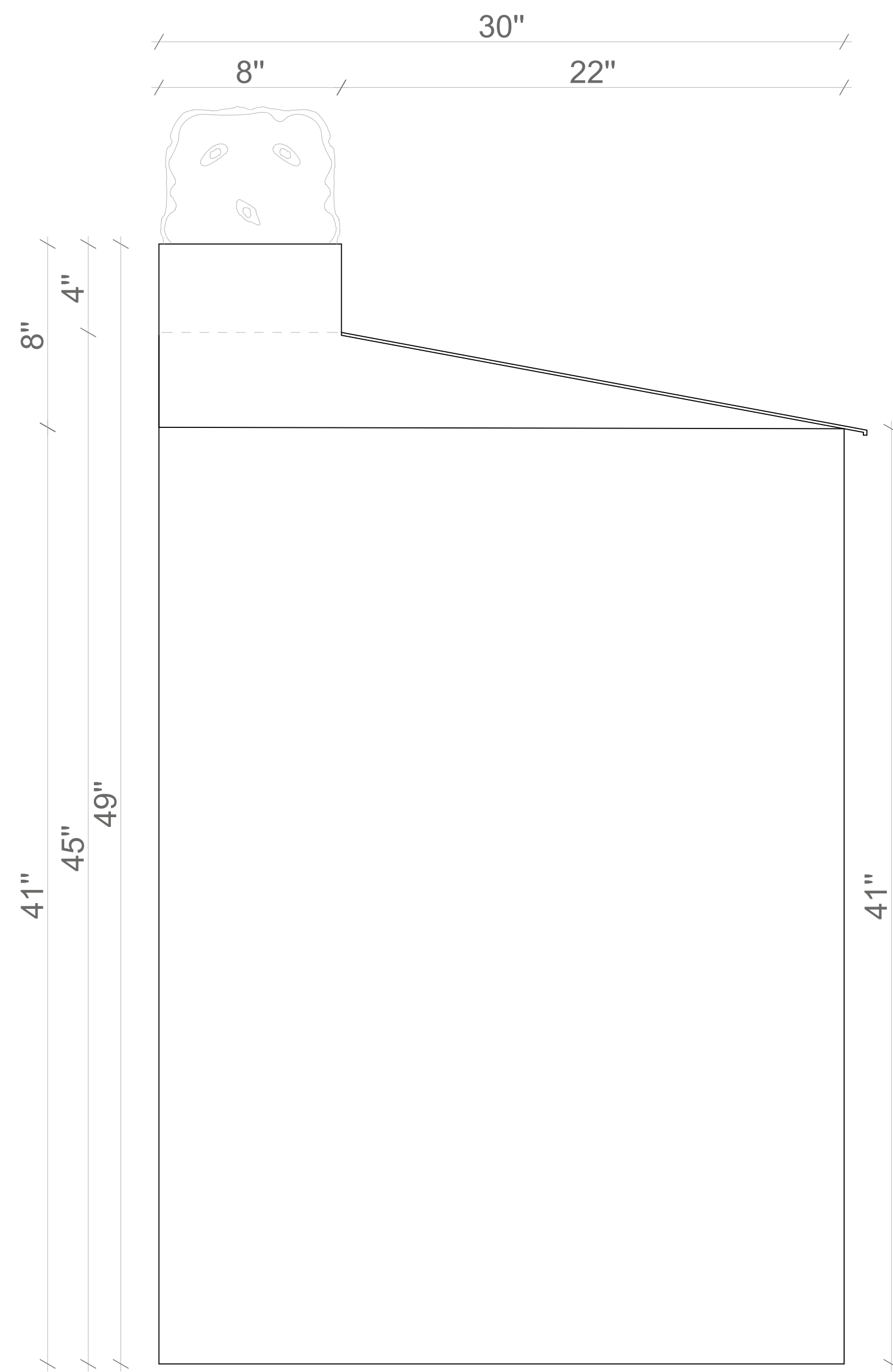
3 GARBAGE SIDE VIEW SCALE: 3" = 1'-0"
