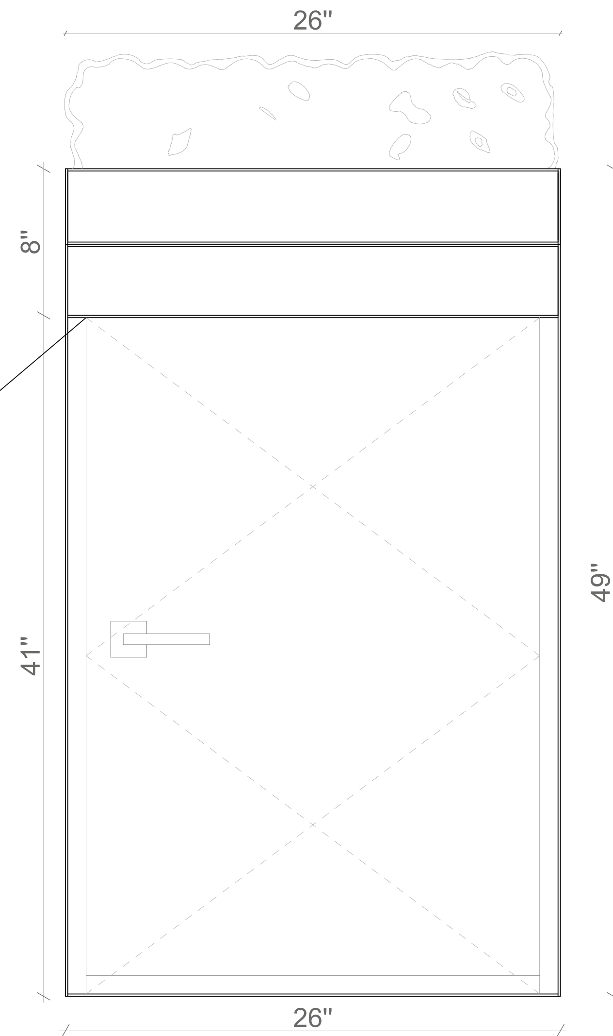
2 GARBAGE FRONT VIEW SCALE: 3" = 1'-0"
