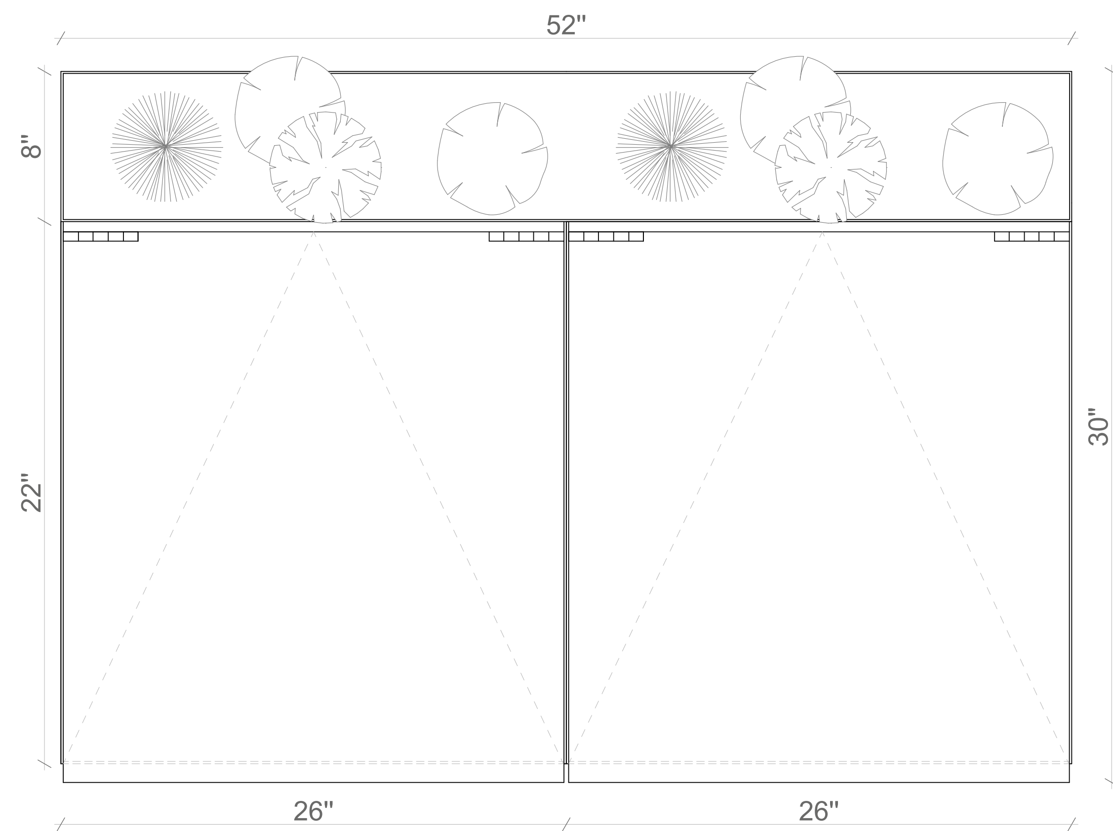
1 GARBAGE TOP VIEW SCALE: 3" = 1'-0"
