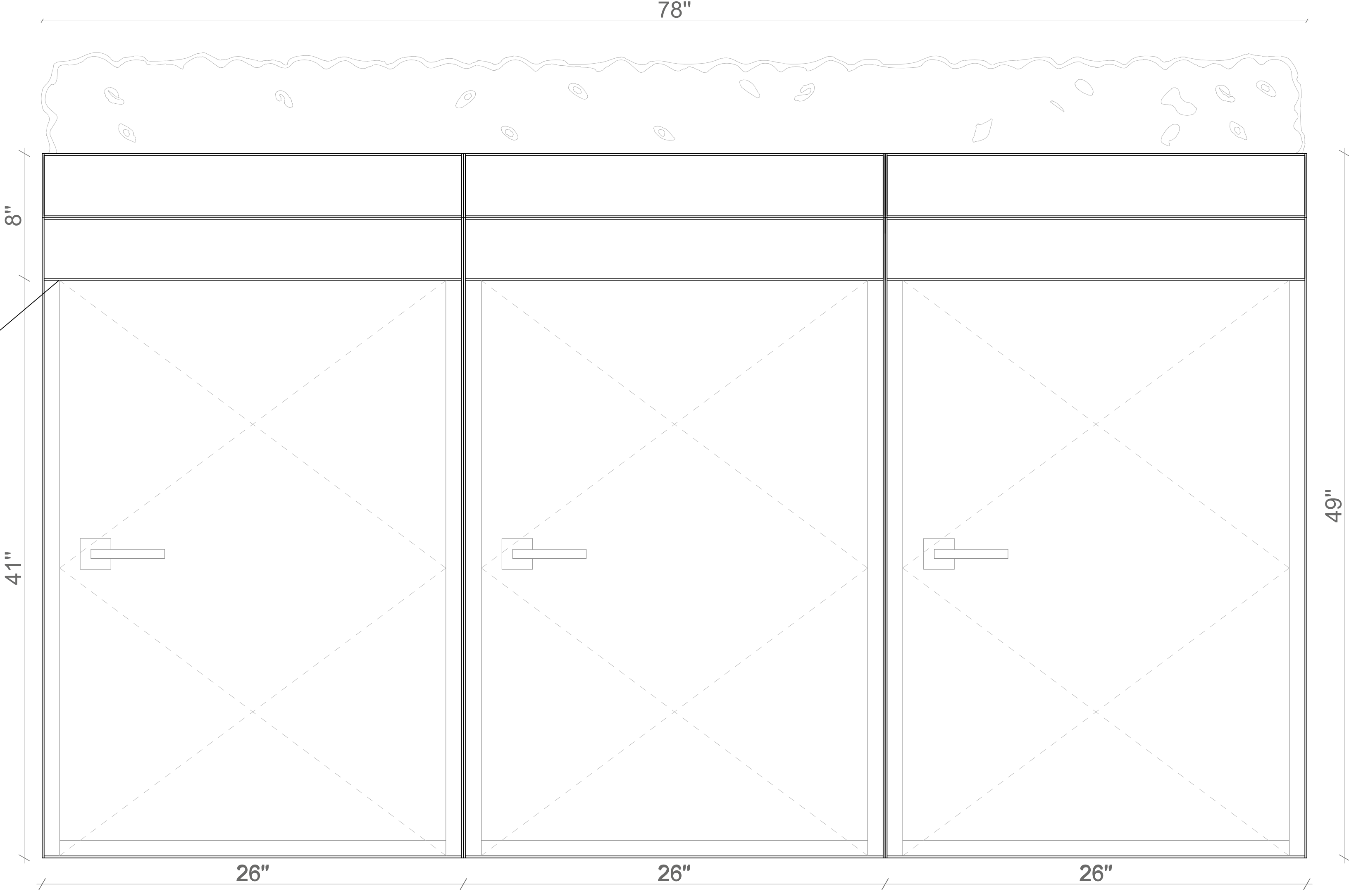
2 GARBAGE FRONT VIEW SCALE: 3" = 1'-0"
